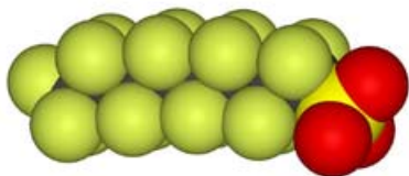
Kalottenmodell des Perfluorooctansulfonats. Links die unpolare perfluorierte Kette; rechts die negativ geladene, polare Sulfonatgruppe. (Quelle: Wikipedia)
